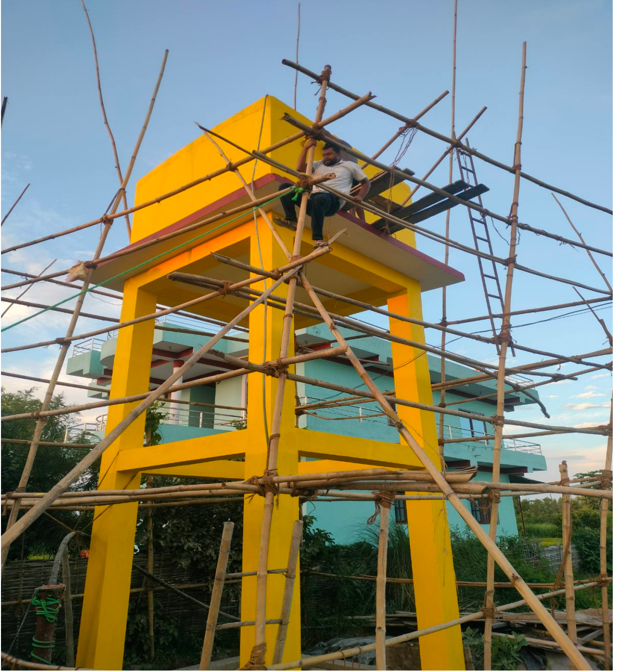
वडा नं १३ स्थित ओभरहेड ट्याङ्की (१८००० लि.)
